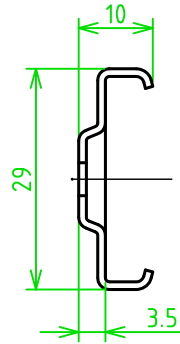
X-X断面拡大図(1/1)
