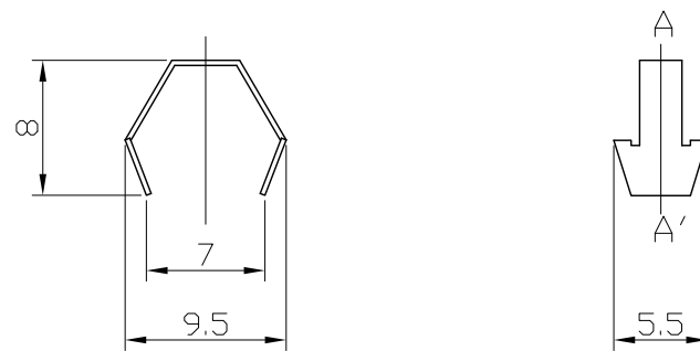
A-A'断面図
