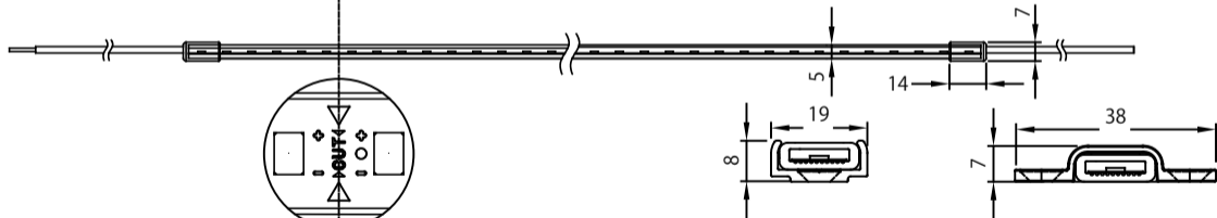
固定具取付図 (1:1) (VB1)
